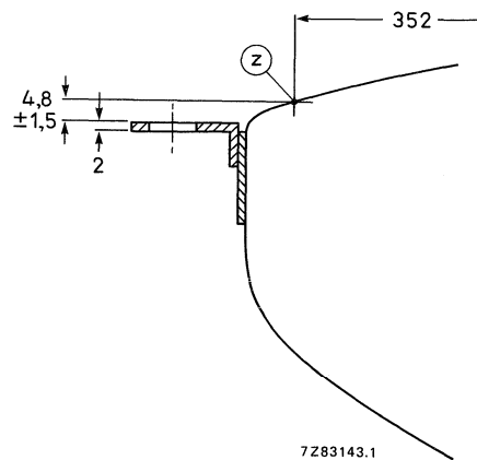
Fig. 15 Lug position.
