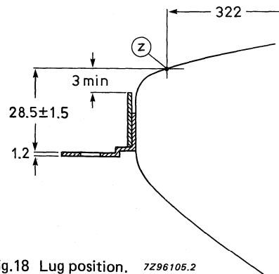
Fig.18 Lug position. 7296105.2
