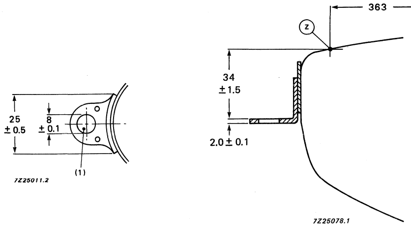
Fig. 15 Lug position.
