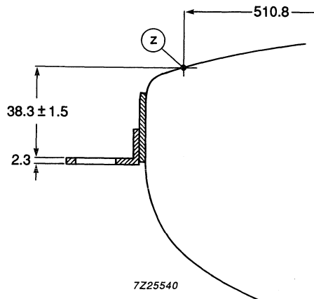
Fig. 15 Lug position.
