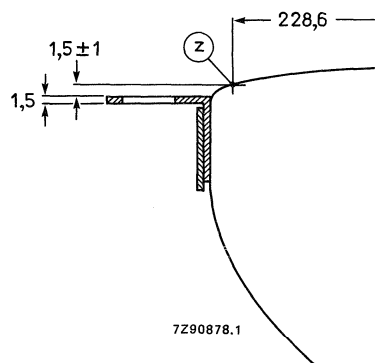
Fig. 13 Lug position.
