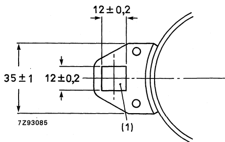
Fig. 17 Lug dimensions.
