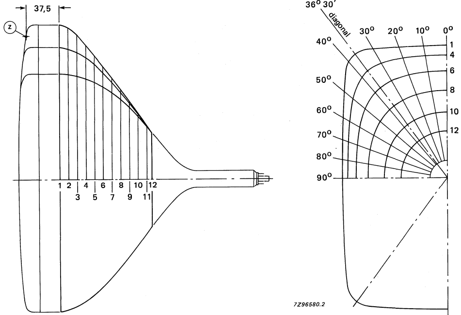
Fig.18 Cone contour.
