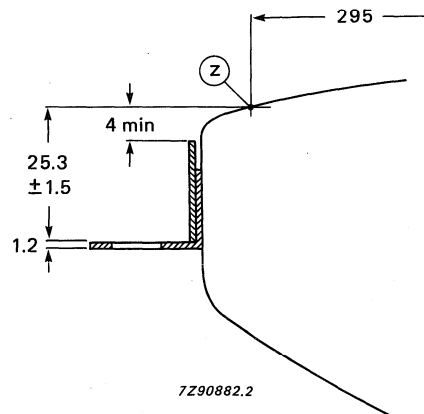
Fig. 15 Lug position.
