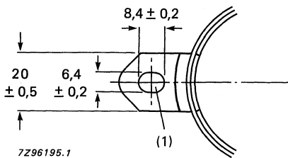
Fig.17 Lug dimensions.
