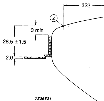
Fig.20 Lug position.
