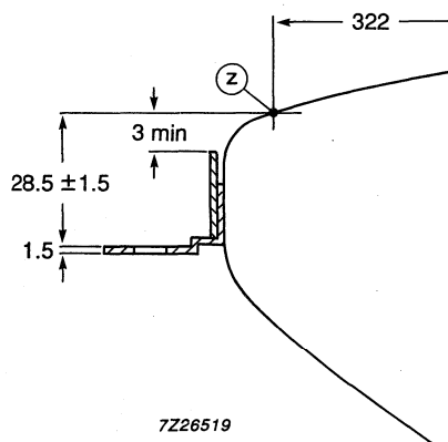
Fig.17 Lug position.
