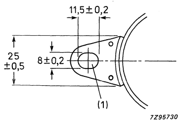
Fig. 14 Lug dimensions.
