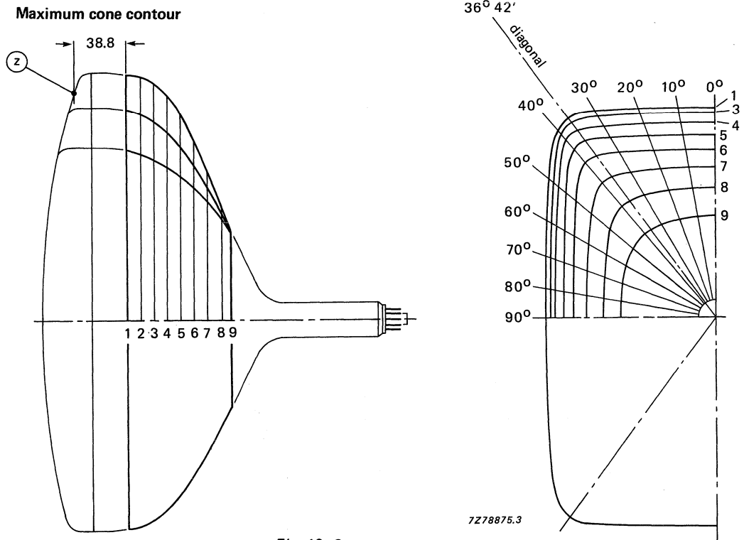
Fig. 19 Cone contour.
