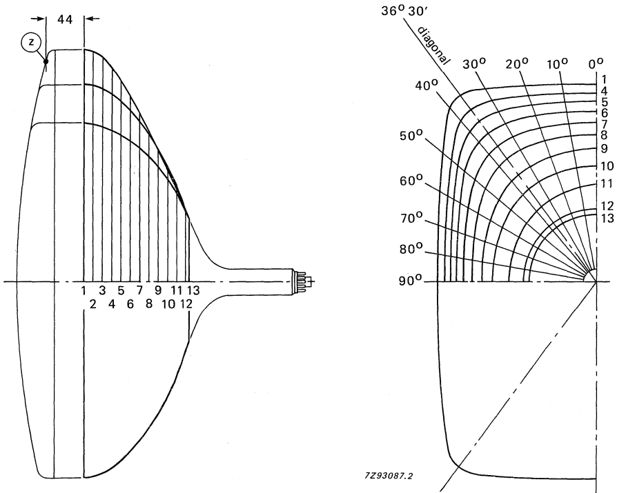
Fig. 19 Cone contour.
