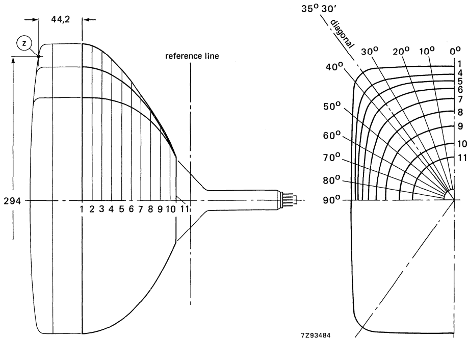
Fig. 18 Cone contour.
