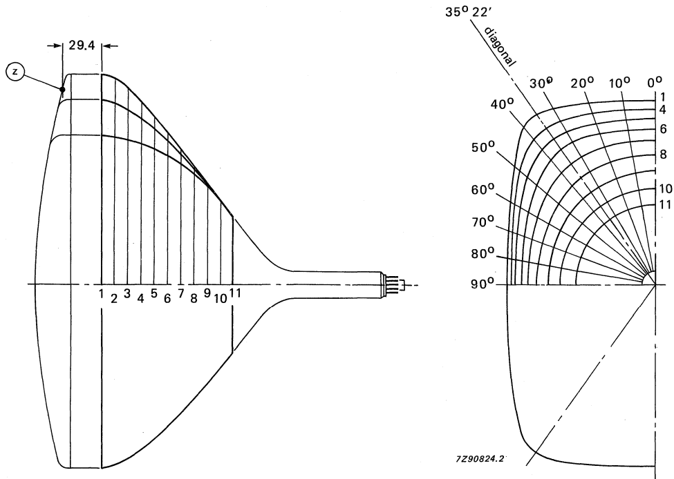
Fig. 21 Cone contour.
