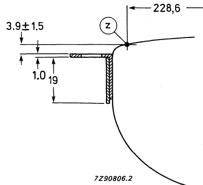
Fig. 18 Lug position.
