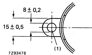
Fig. 16 Lug position.
