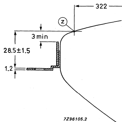
Fig.17 Lug position.
