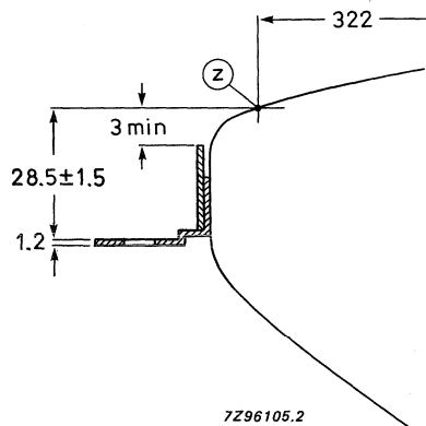
Fig.15 Lug position.
