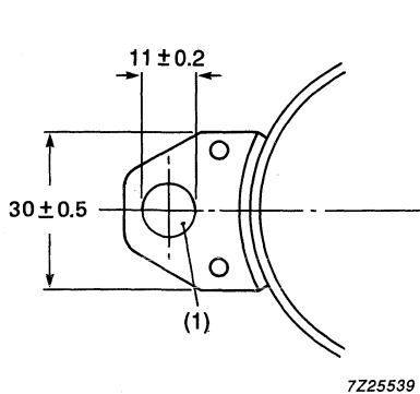
Fig. 14 Lug dimensions.
