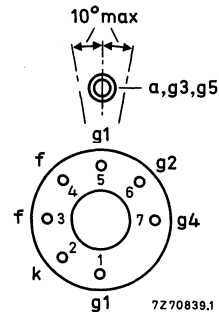
Fig. 12 Pin arrangement.
