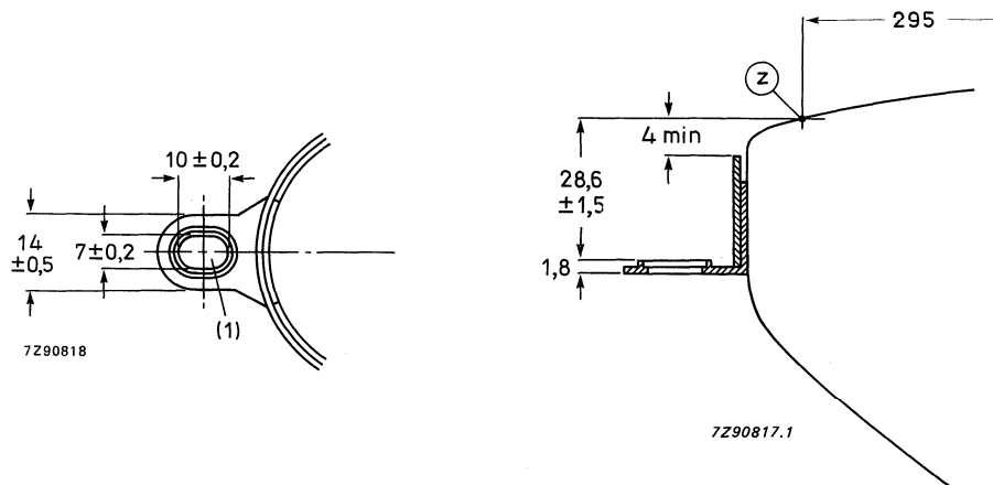
Fig. 22 Lug dimensions.
