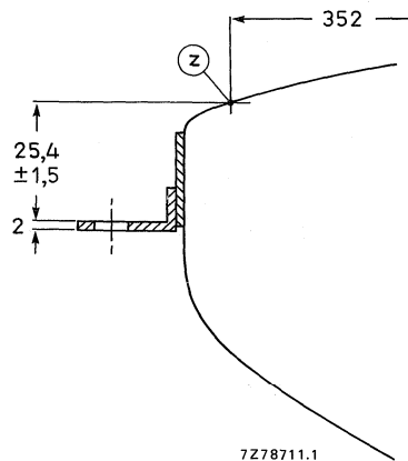
Fig. 15 Lug position.
