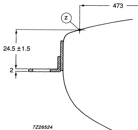
Fig. 18 Lug position.
