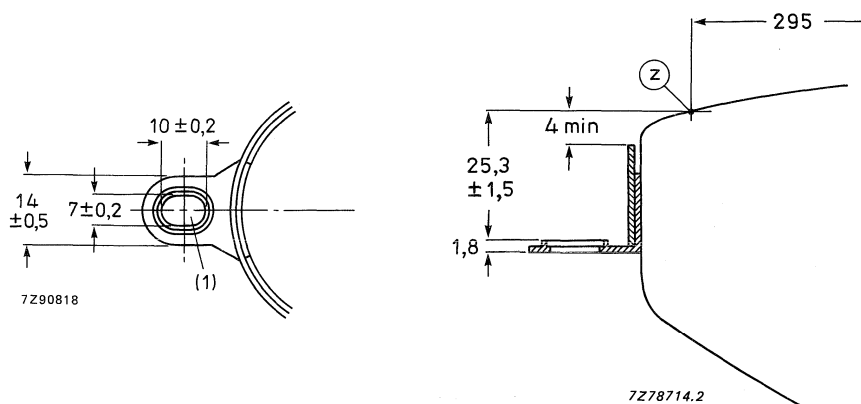
Fig. 14 Lug dimensions.
