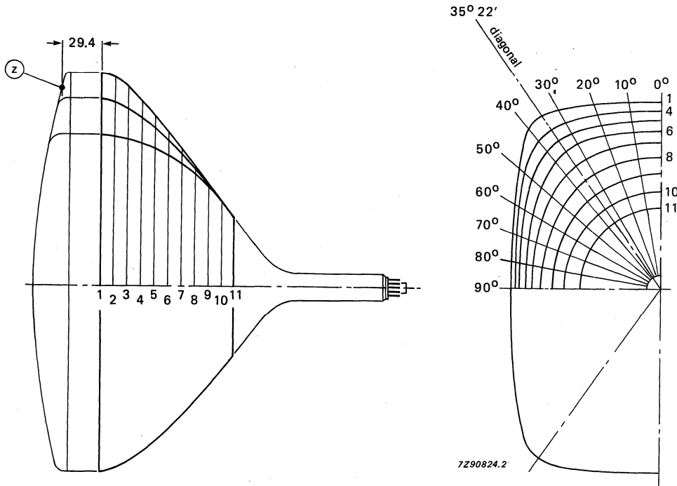
Fig. 16 Cone contour.
