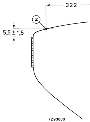
Fig.14 Lug position.
