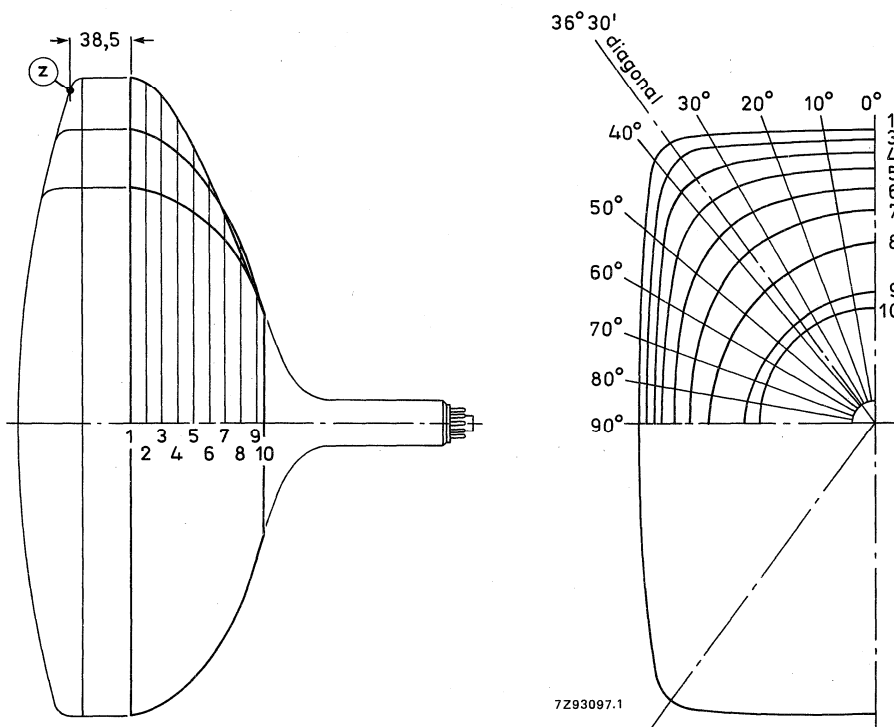
Fig. 16 Cone contour.
