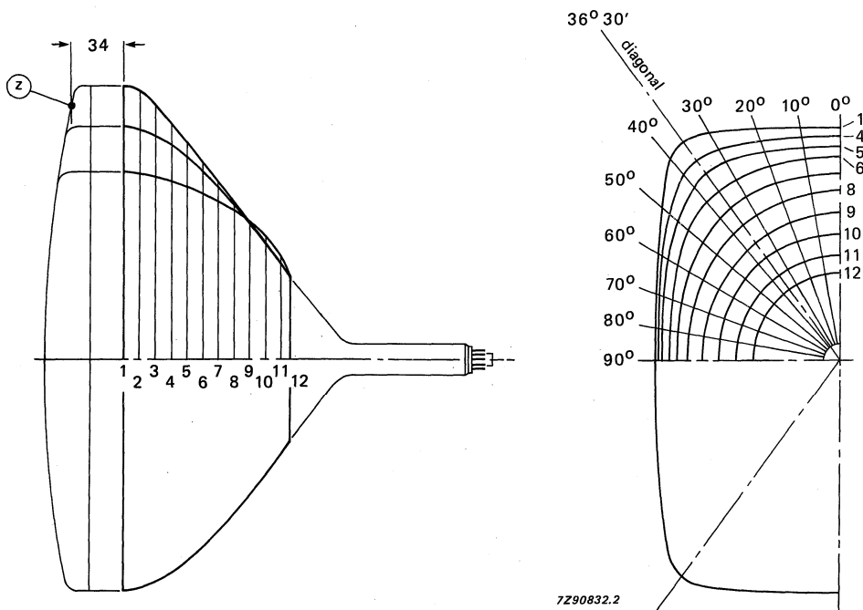
Fig.18 Cone contour.
