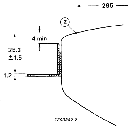
Fig. 26 Lug position.
