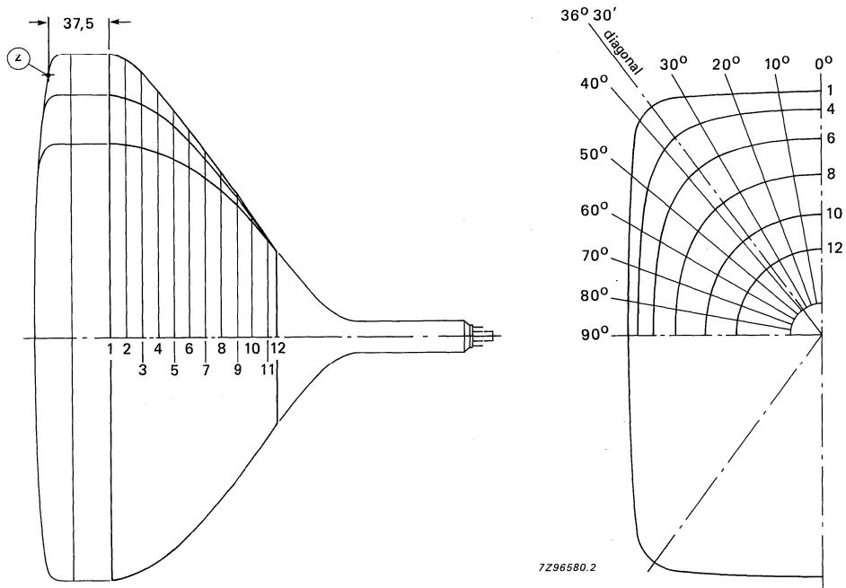
Fig.18 Cone contour.
