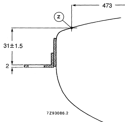
Fig. 15 Lug position.
