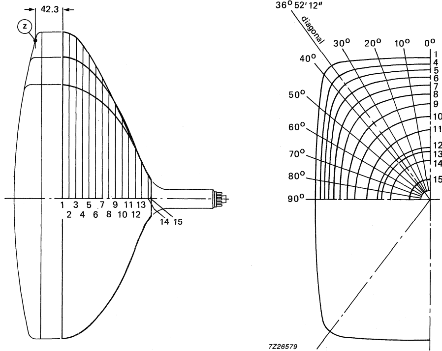
Fig. 16 Cone contour.
