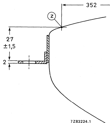
Fig. 21 Lug position.
