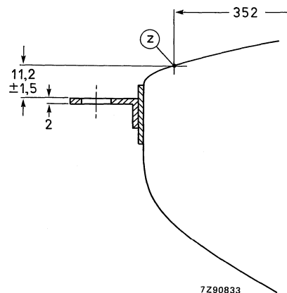
Fig. 24 Lug position.
