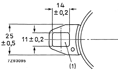
Fig. 14 Lug dimensions.
