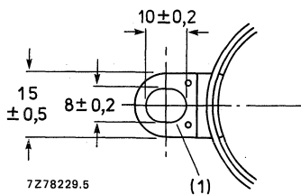
Fig. 14 Lug dimensions.
