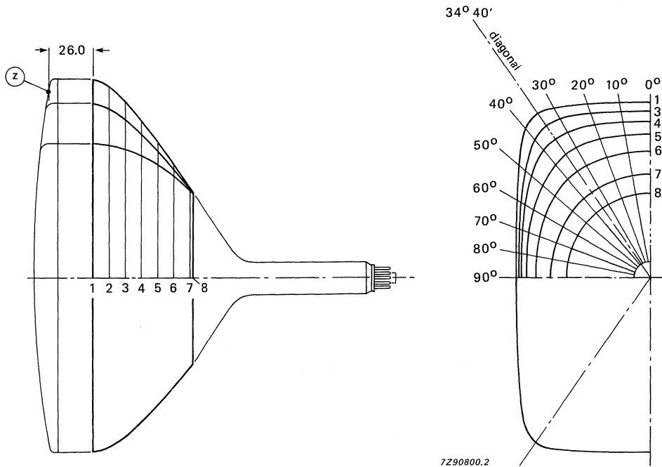
Fig. 19 Cone contour.
