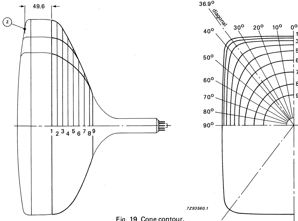
Fig. 19 Cone contour.
