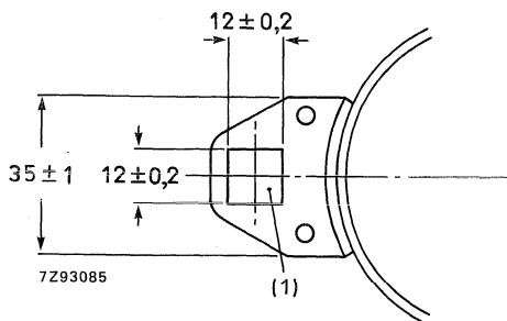
Fig. 14 Lug dimensions.
