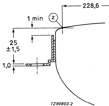
Fig. 15 Lug position.
