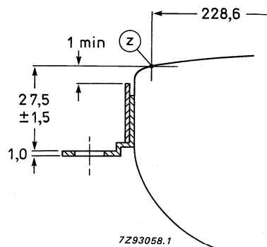
Fig. 24 Lug position.
