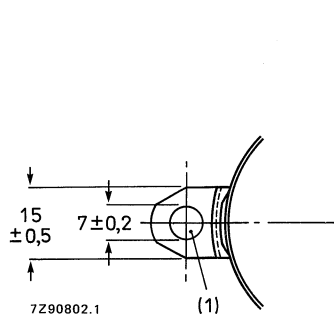
Fig. 23 Lug dimensions.
