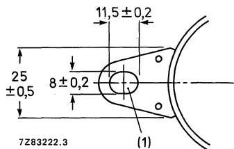
Fig. 23 Lug dimensions.
