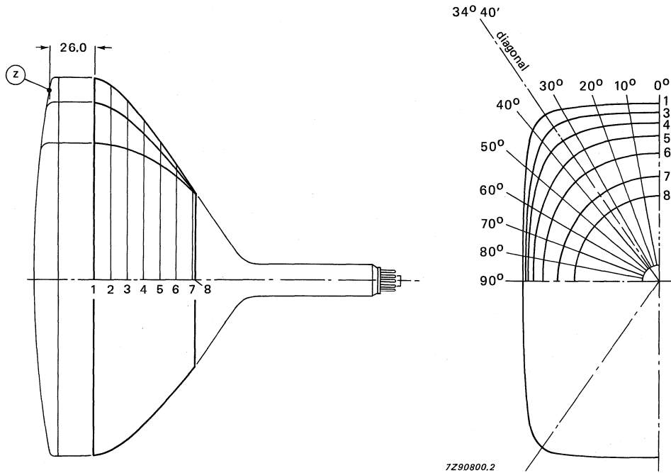
Fig. 14 Cone contour.
