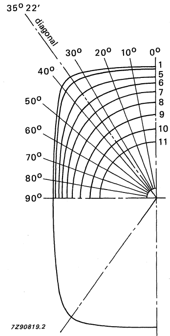
Fig. 22 Cone contour.
