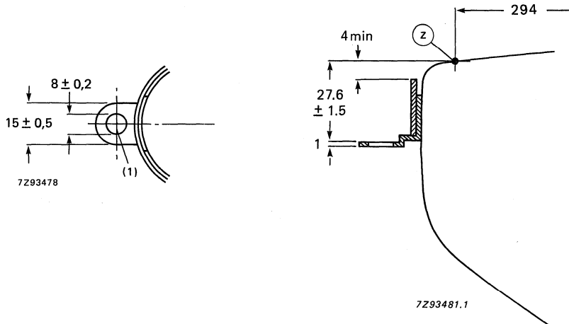
Fig. 16 Lug dimensions.
