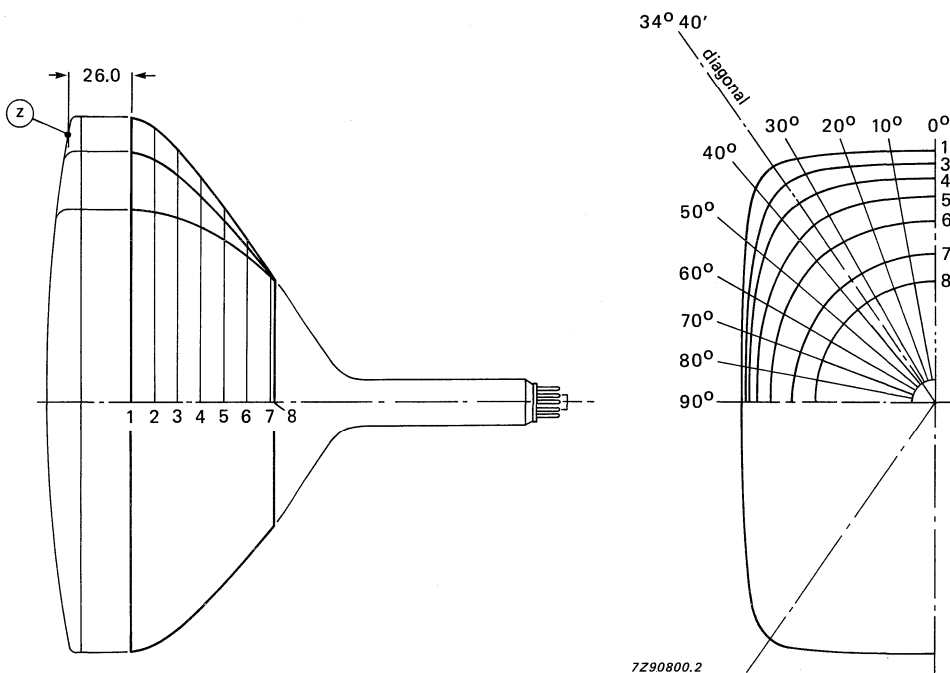
Fig. 25 Cone contour.
