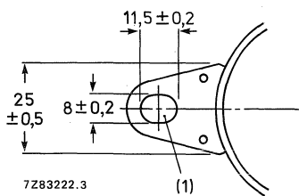
Fig. 14 Lug dimensions.
