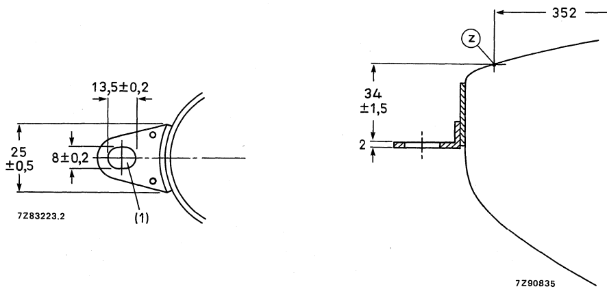
Fig. 29 Lug dimensions
