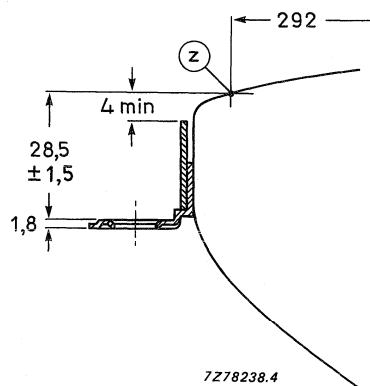
Fig. 15 Lug position.
