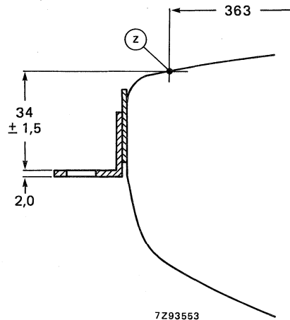
Fig. 18 Lug position.
