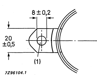
Fig.16 Lug dimensions.
