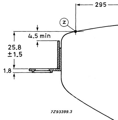
Fig. 21 Lug position.
