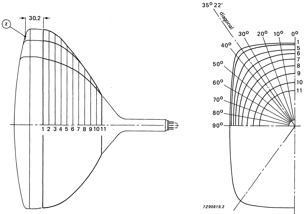
Fig. 27 Cone contour.
