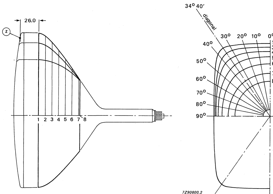
Fig. 16 Cone contour.
