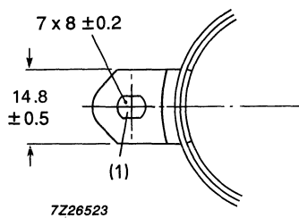
Fig.19 Lug dimensions.
