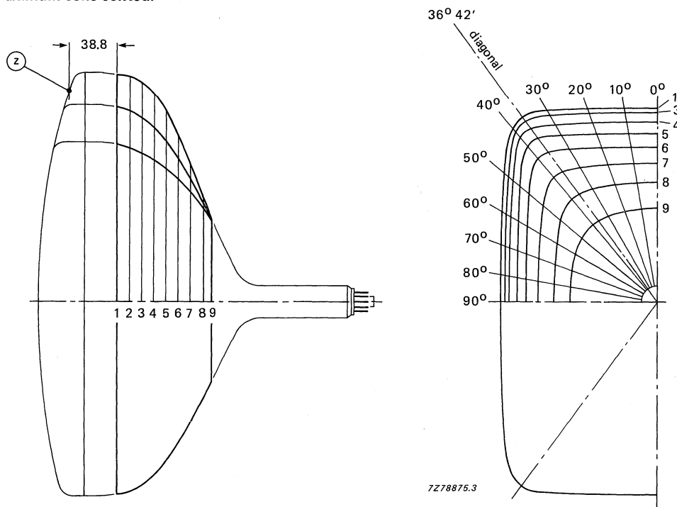
Fig. 31 Cone contour.
