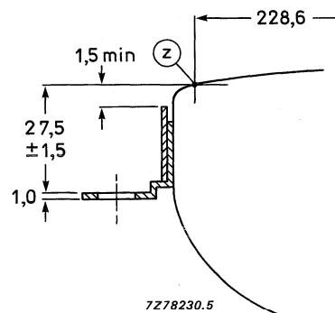
Fig. 15 Lug position.
