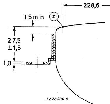
Fig. 15 Lug position.
