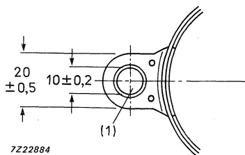
Fig. 14 Lug dimensions.
