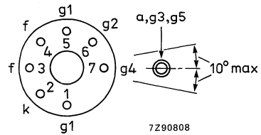
Fig. 10 Pin arrangement.
