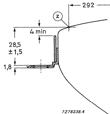
Fig. 15 Lug position.
