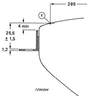
Fig. 15 Lug position.
