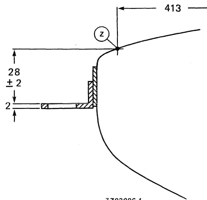
7293096.1 Fig. 15 Lug position.
