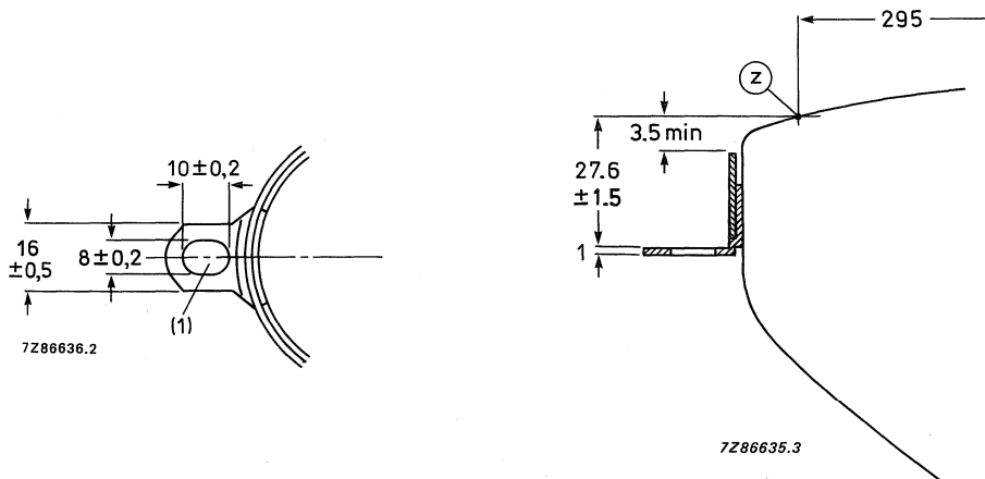
Fig. 17 Lug dimensions.
