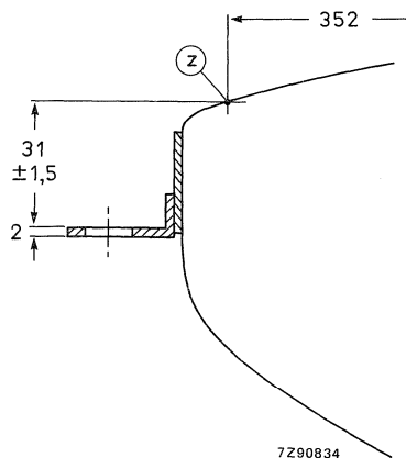
Fig. 27 Lug position.
