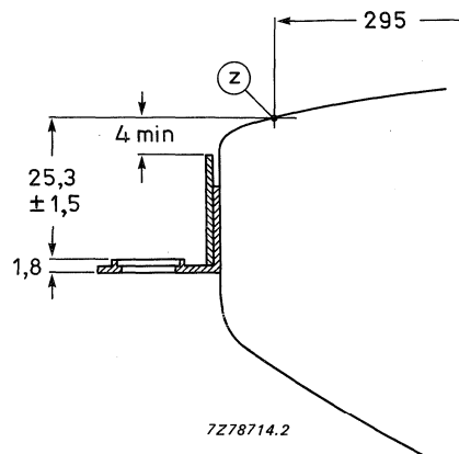
Fig. 15 Lug position.
